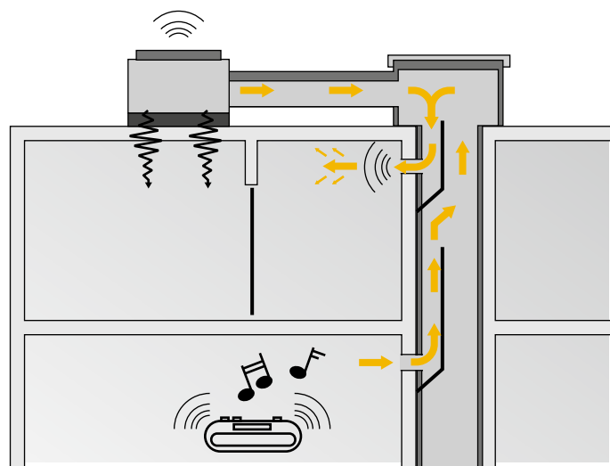
Figure 10 : Sources sonores transmises par l'installation de ventilation
