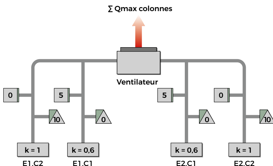
Figure B.3 – Schéma du réseau d'extraction par colonne
