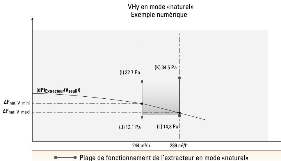
Figure D.8 – Exemple numérique de dimensionnement de l'extracteur en mode « naturel »
