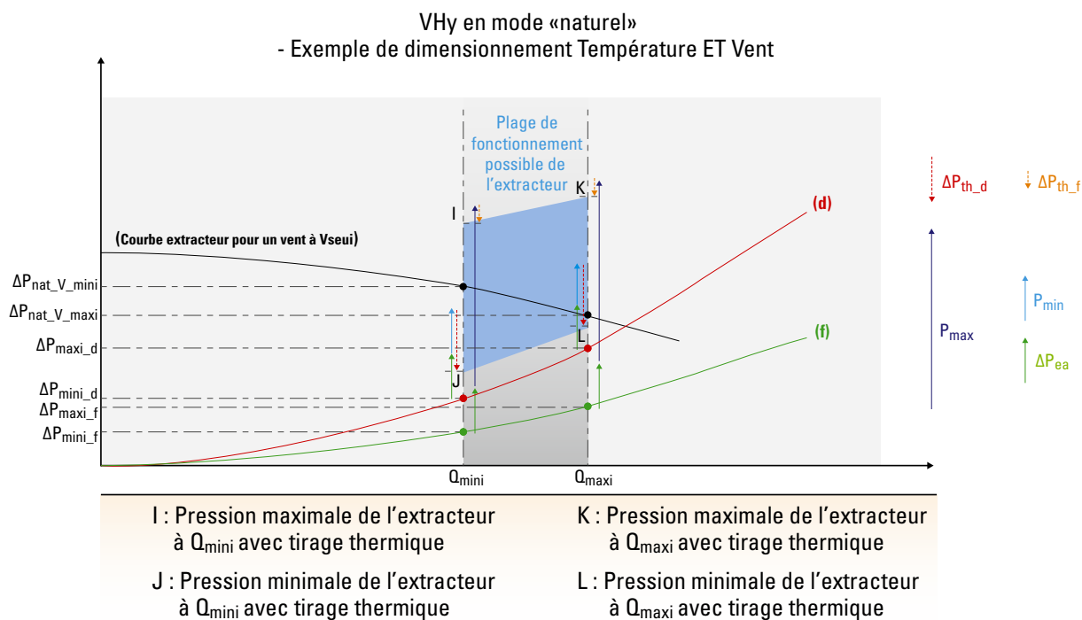
Figure D.5 – Illustration du dimensionnement de l'extracteur en mode « naturel »
