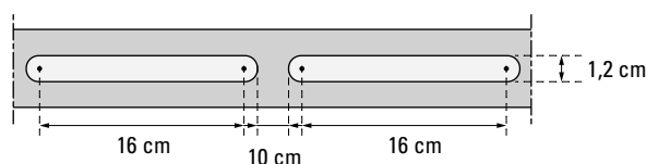
Figure 12 : Exemple de dimensions des réservations pour la pose d'entrées d'air sur menuiserie, mortaise après 1999
