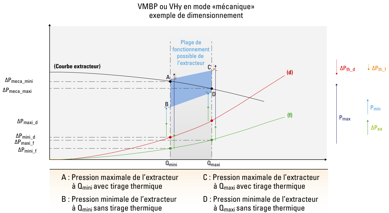
Figure D.1 – Illustration du dimensionnement de l'extracteur en mode « mécanique »
