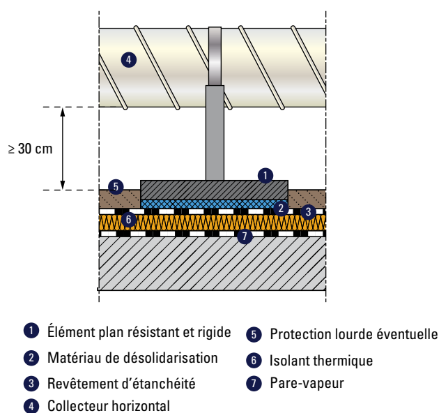
Figure 25 : Supports de collecteurs en terrasse
