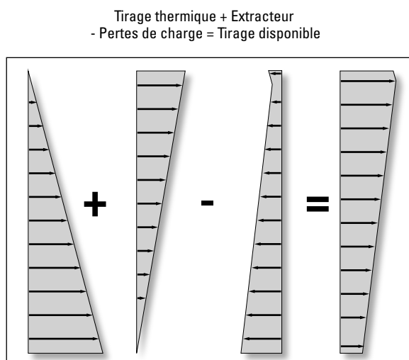
Figure 7 : Equilibre des forces et point de fonctionnement de l'installation
