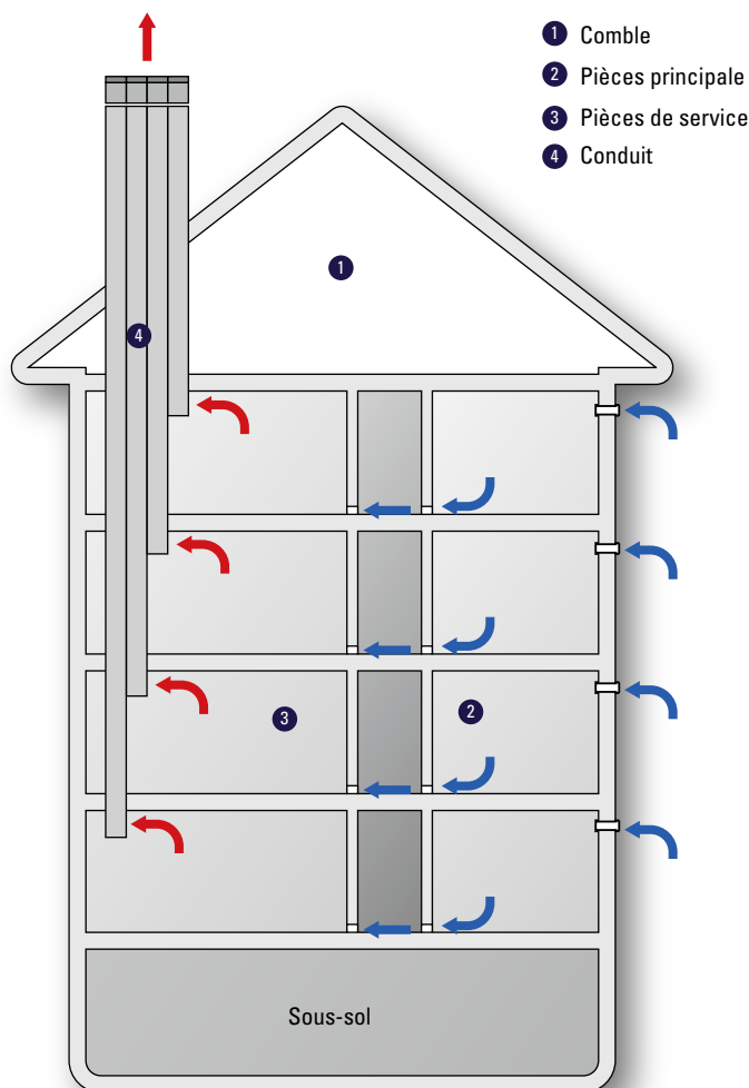
Figure 3 : Configuration de conduits individuels
