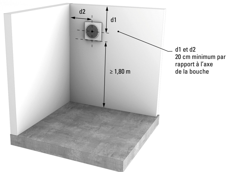
Figure 13 : Emplacement des bouches (cas de création de conduit neuf)
