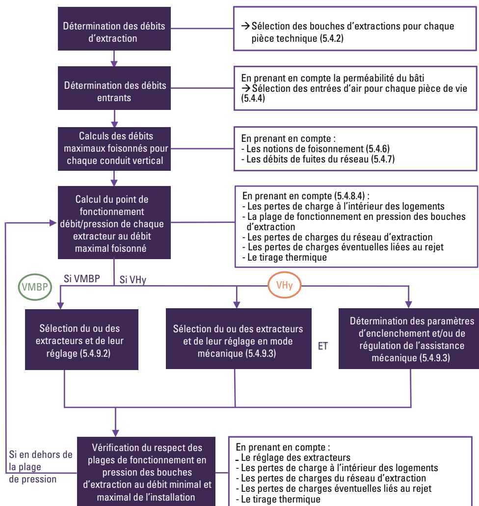
Figure 8 : Fil conducteur de la conception
