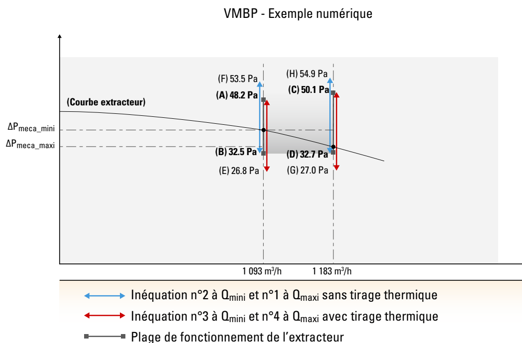
Figure D.4 – Exemple numérique de dimensionnement de l'extracteur en mode « mécanique »
