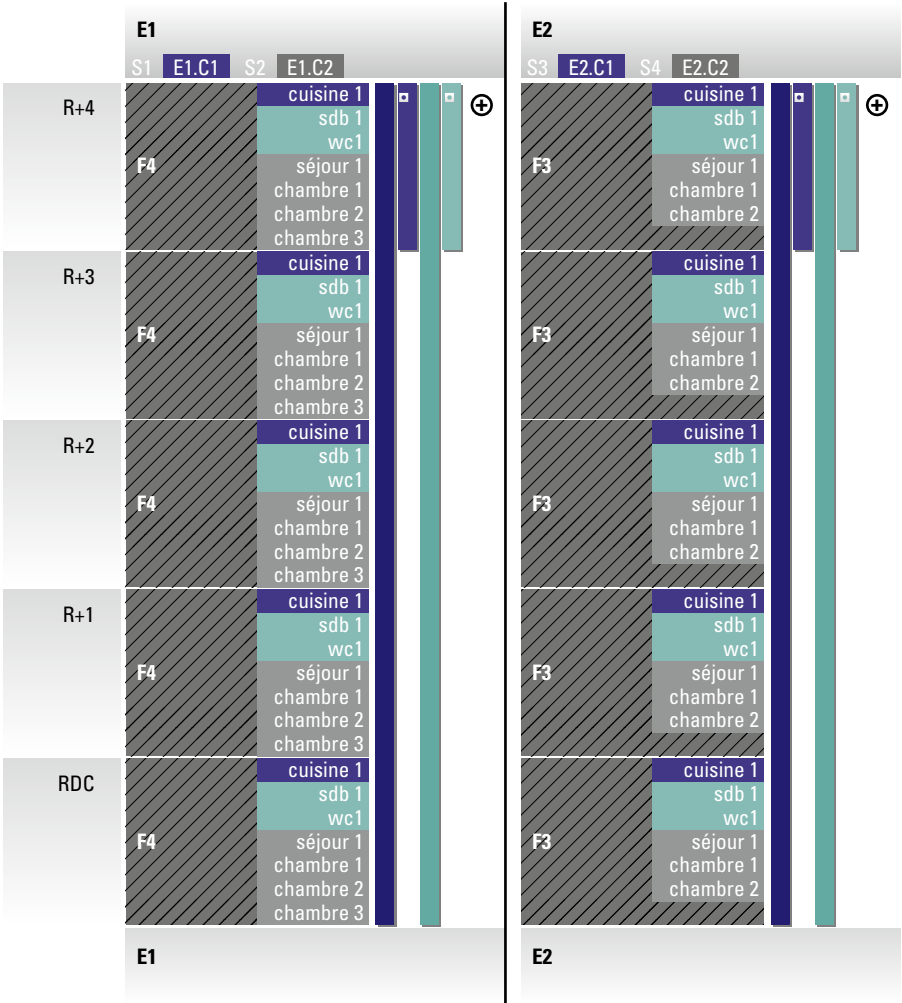
Figure D.2 – Plan d'élévation du bâtiment avec représentation schématique des conduits verticaux
