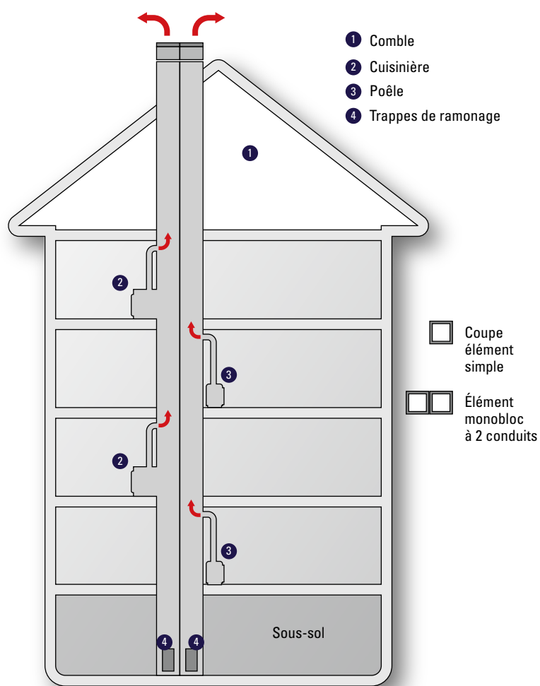
Figure 4 : Configuration de conduits Alsace
