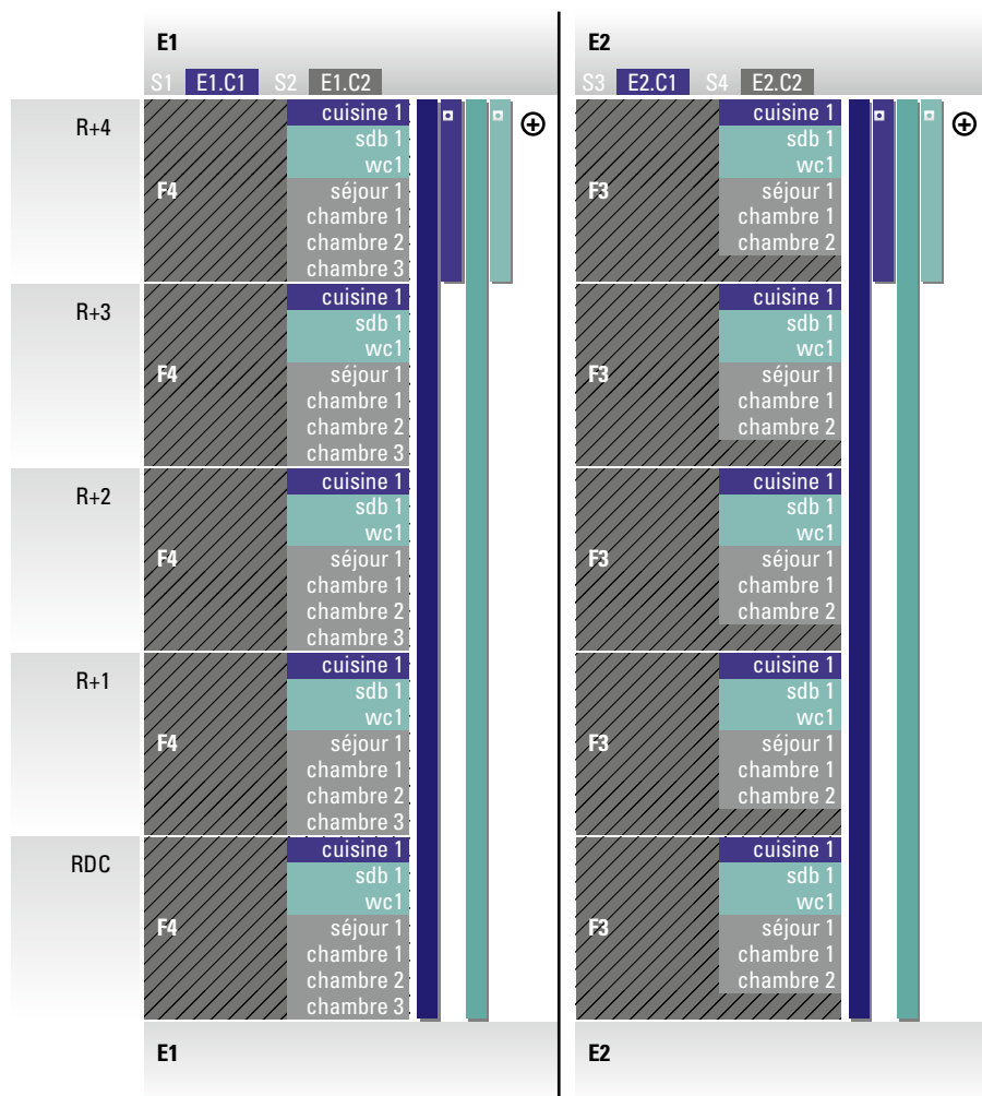
Figure B.2 – Plan d'élévation du bâtiment avec représentation schématique des conduits verticaux
