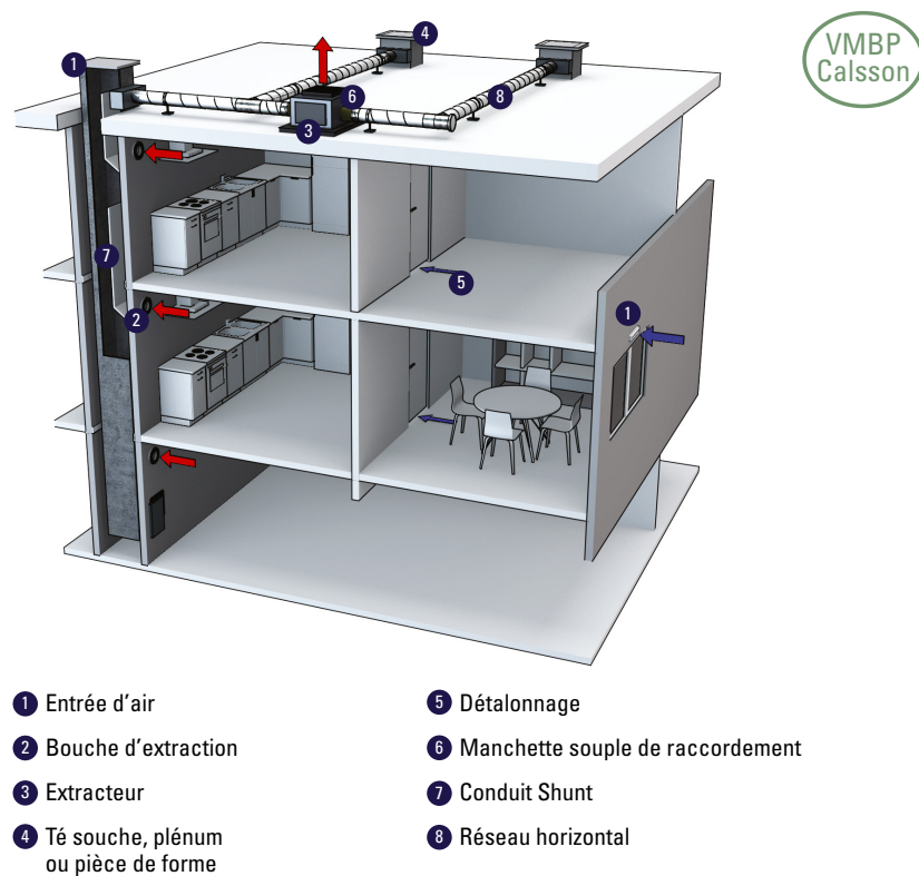
Figure 1 : Schéma type d'une installation en ventilation mécanique basse pression (VMBP) avec réseau en terrasse
