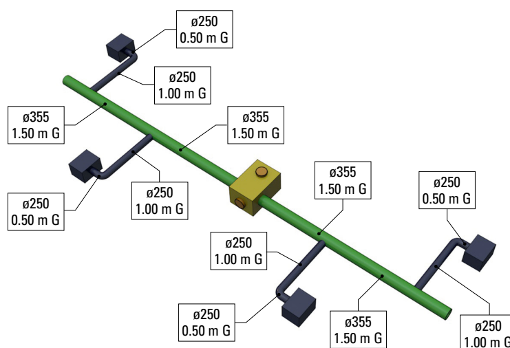
Figure D.3 – Schéma du réseau terrasse neuf
