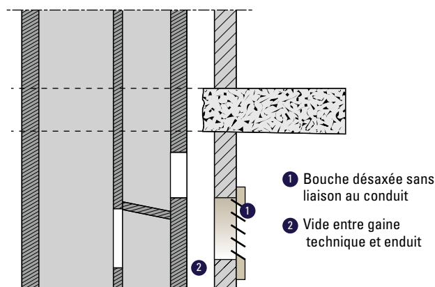
Figure 14 : Exemples de défauts de liaison entre conduit et cloison
