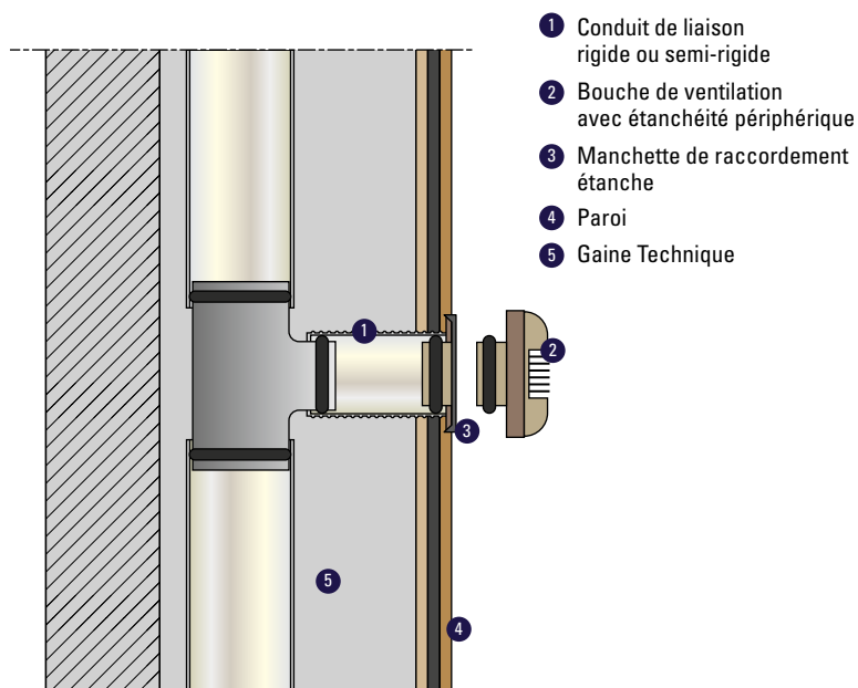
Figure 17 : Jonction entre le dispositif d'extraction et le conduit de liaison avec manchette de raccordement
