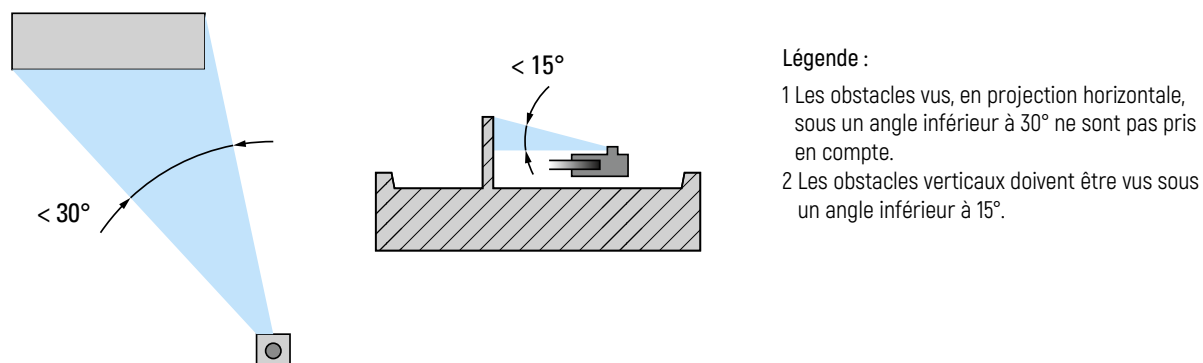
Figure 29 : Règle de calcul des distances minimales entre l'orifice de rejet et les obstacles en toiture
