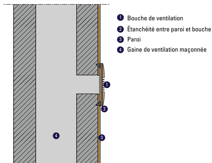
Figure 15 : Bouche en applique sur conduit maçonné
