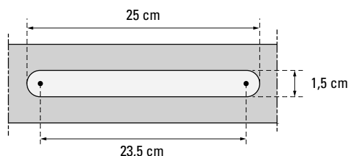
Figure 11 : Exemple de dimensions des réservations pour la pose d'entrées d'air sur menuiserie, mortaise avant 1999
