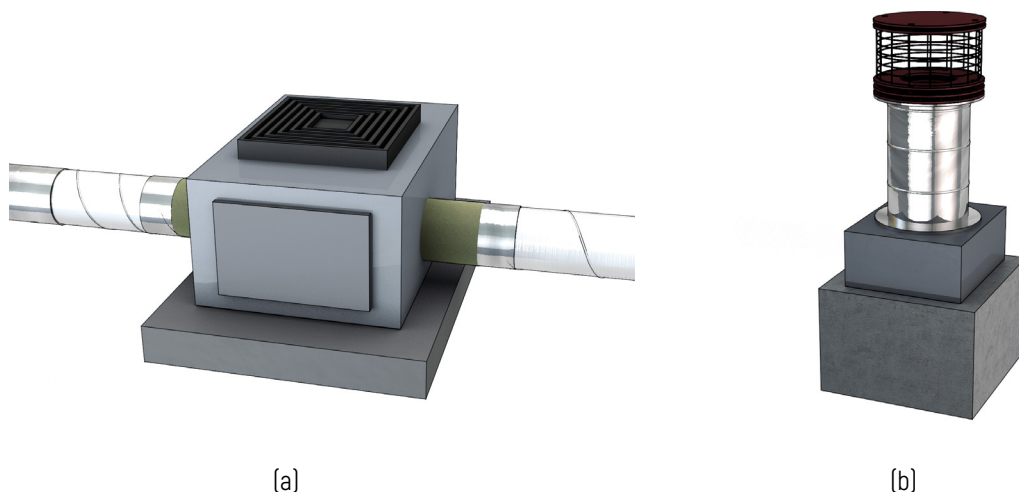
Figure 9 : Rejet d'air dirigé vers le haut (a) ou dans une couronne à 360° d'axe vertical (b)
