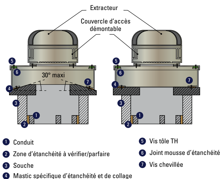
Figure 33 : Vue en coupe d'un extracteur avec plenum fixé sur conduit existant et dalle conservée
