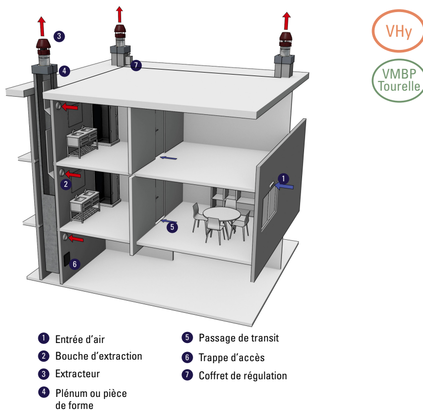
Figure 2 : Schéma type d'une installation en ventilation mécanique basse pression (VMBP) ou en ventilation hybride (VHy) avec extracteur en débouché de conduit
