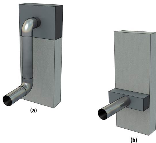
Figure 19 : Exemples de plenums (a) plenum de recouvrement (b) plenum en piquage
