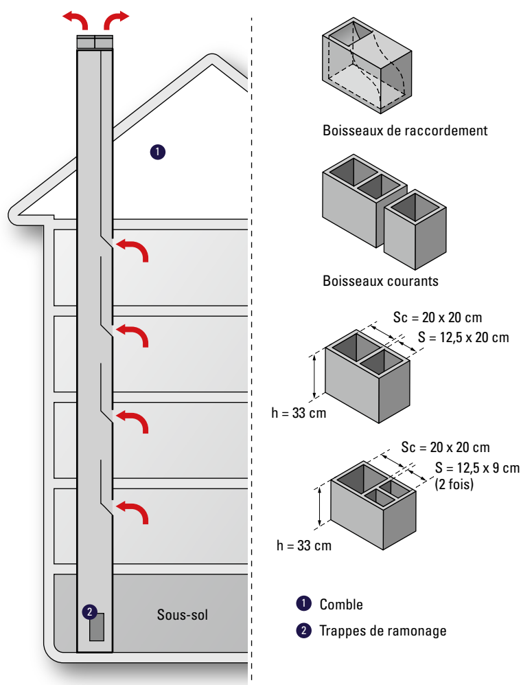
Figure 5 : Configuration de conduits dits « Shunt »
