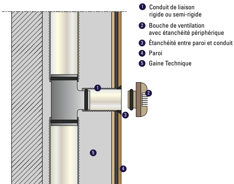
Figure 18 : Jonction entre le dispositif d'extraction et le conduit de liaison sans manchette de raccordement
