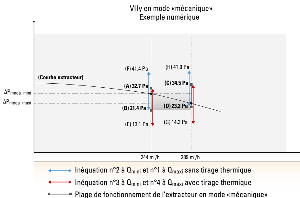
Figure D.7 – Exemple numérique de dimensionnement de l'extracteur en mode « mécanique »
