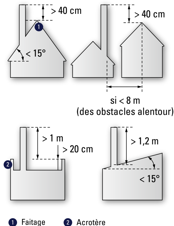
Figure 34 : Dispositions à respecter pour le positionnement des rejets d'air en toiture
