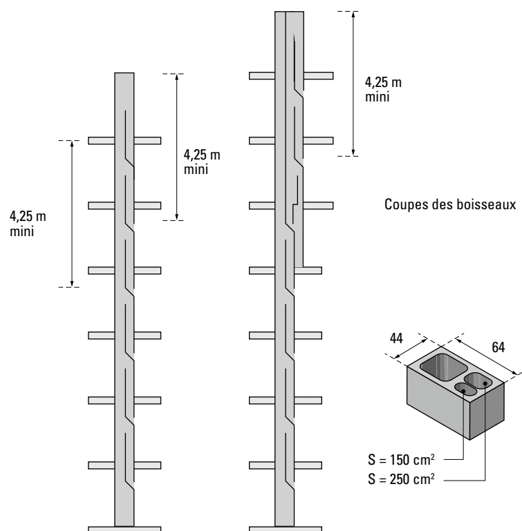
Figure 6 : Configurations de conduits mixtes
