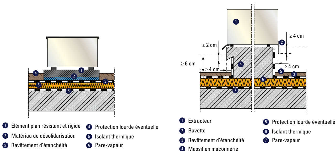
Figure 26 et 27 : Exemple de pose de l'extracteur en terrasse [solution 1 et solution 2]
